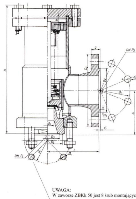
ZAWORY BEZPIECZEŃSTWA ZBKk 32÷50
