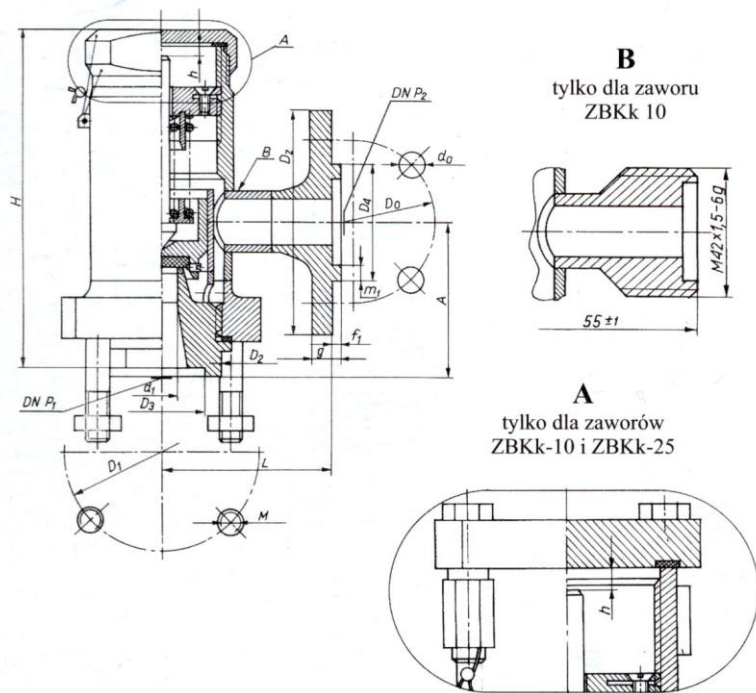
ZAWORY BEZPIECZEŃSTWA ZBKk 10÷25
